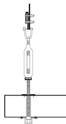
EJEMPLO DE SISTEMA DE CUELQUE A TECHO
