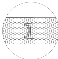
DETALLE JUNTA UNIÓN PANEL
